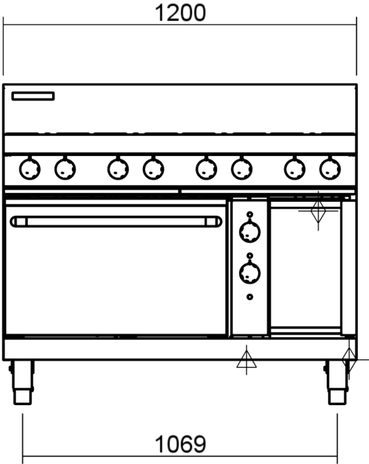
Dimensions GE508 / GE58
